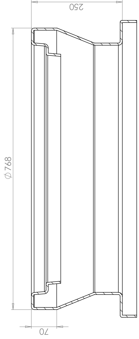
SECTION A-A SCALE 1 : 5
