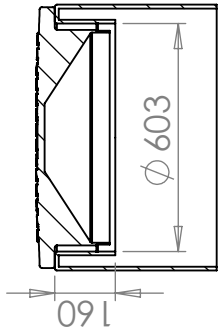
SECTION D-D SCALE 1 : 20
