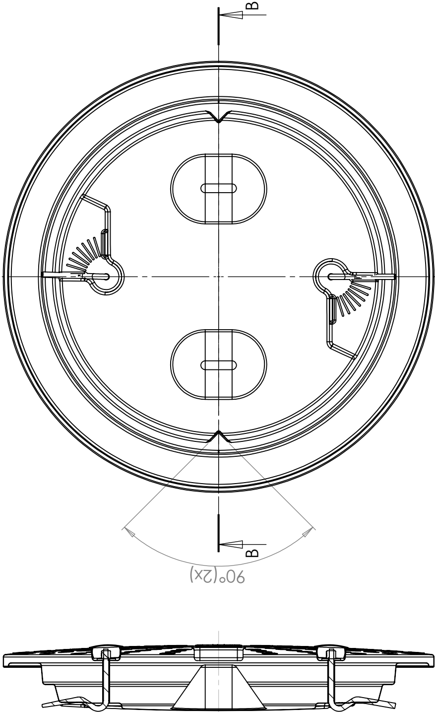
SECTION A-A
