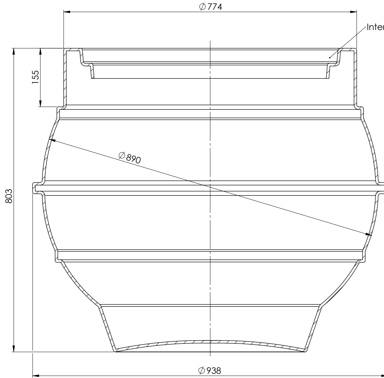
SECTION B-B SCALE 1 : 5
