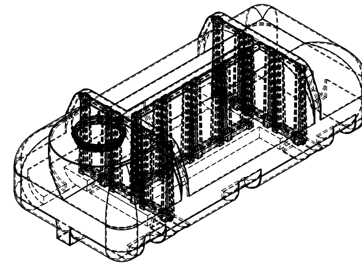
21101 - CPX Beholder 11 000 liter rektangulær 10 skott Mannehull 600 mm. Med 10 innvendige vegger.
