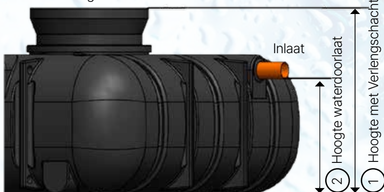
Verlengschacht
